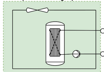
Prinzipdarstellung Hydraulik/Wasserseite
